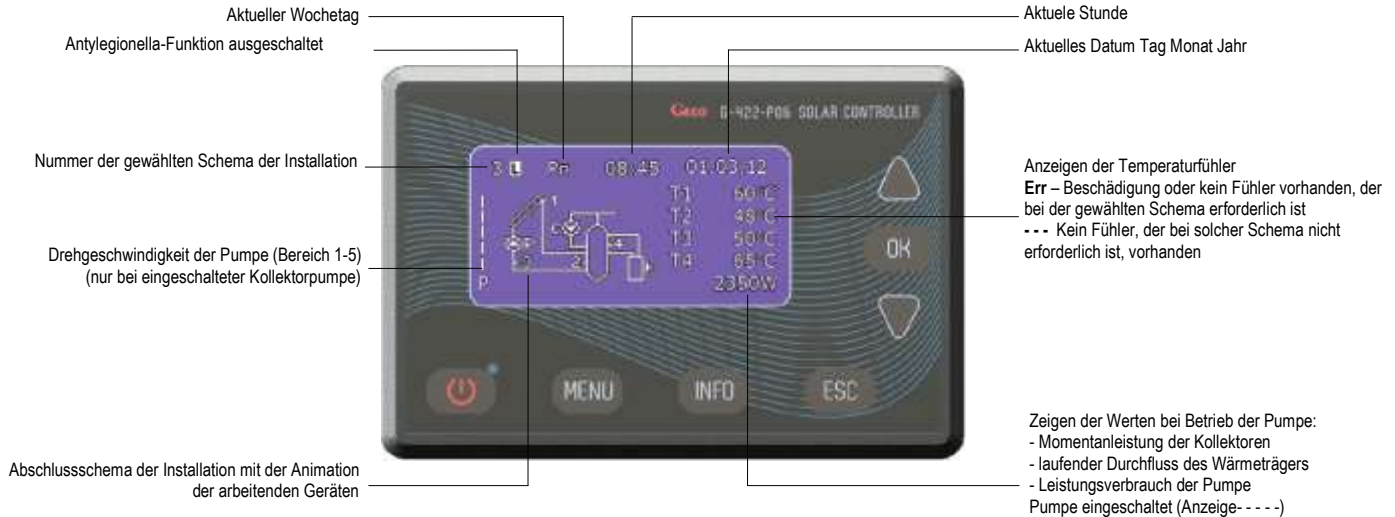
Abb. 2. Beschreibung des Hauptbildschirmes auf dem LCD-Display
