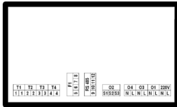
Abb. 1. Kennzeichnung der Eingängen und Ausgängen des Controllers.
