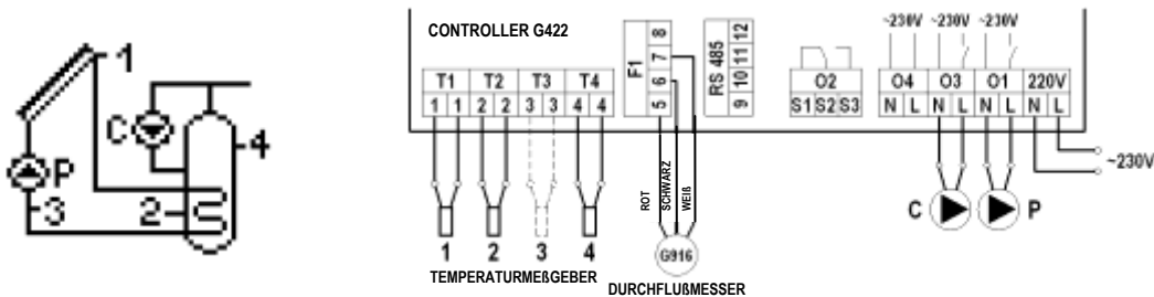
Abb. 4. Anschluss- und elektrisches Schema der Installation 2.
