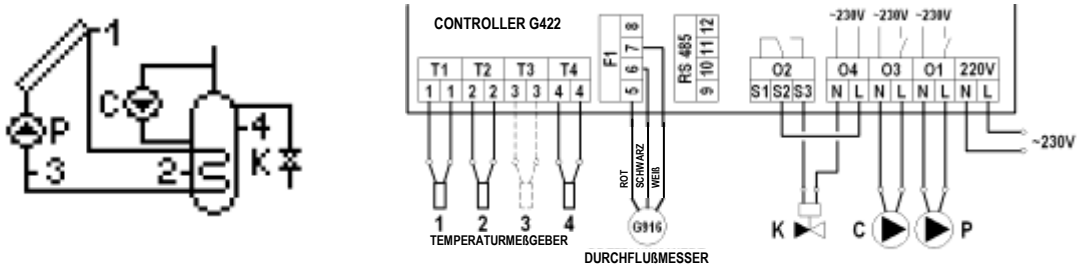
Abb. 19. Anschluss- und elektrisches Schema der Installation Nr. 17.
