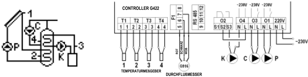
Abb. 8. Anschluss- und elektrisches Schema der Installation 6.
