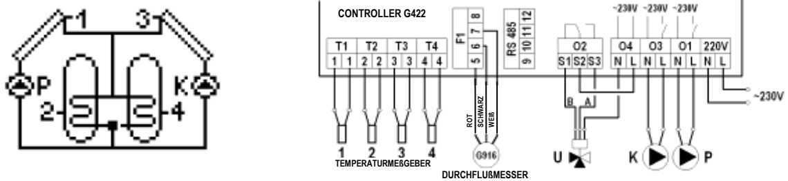
Abb. 18. Anschluss- und elektrisches Schema der Installation 16.
