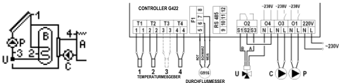
Abb. 11. Anschluss- und elektrisches Schema der Installation 9.
