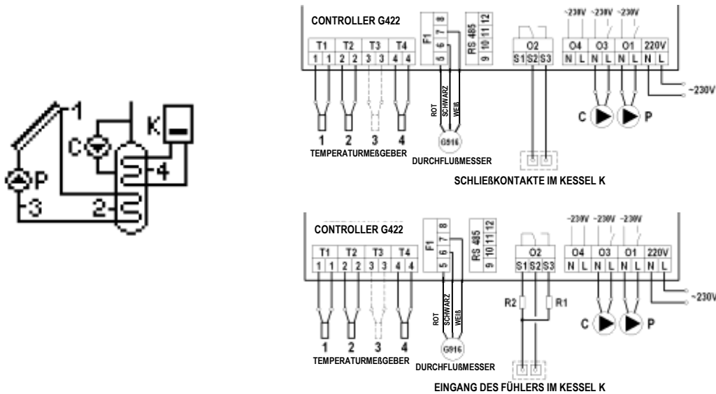
Abb. 5. Anschluss- und elektrisches Schema der Installation 3.
