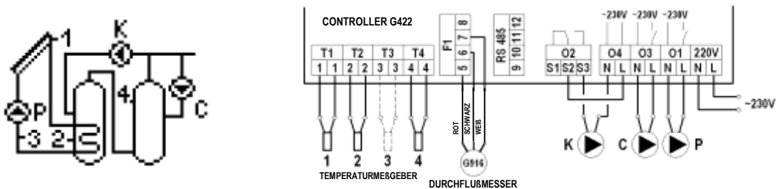
Abb. 9. Anschluss- und elektrisches Schema der Installation 7.
