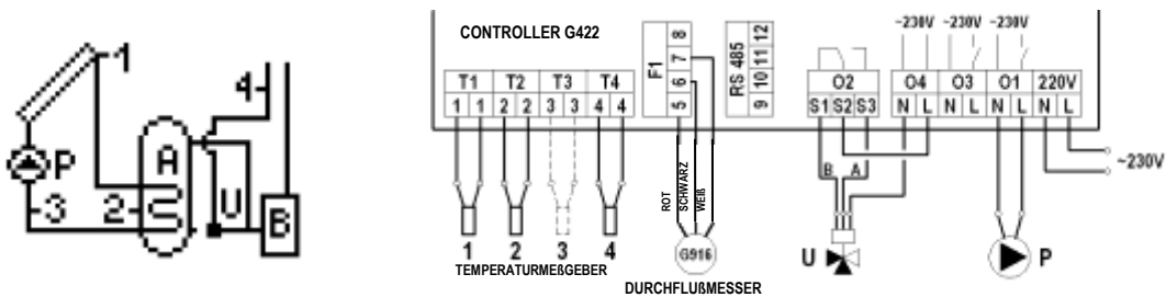
Abb. 15. Anschluss- und elektrisches Schema der Installation Nr. 7.
