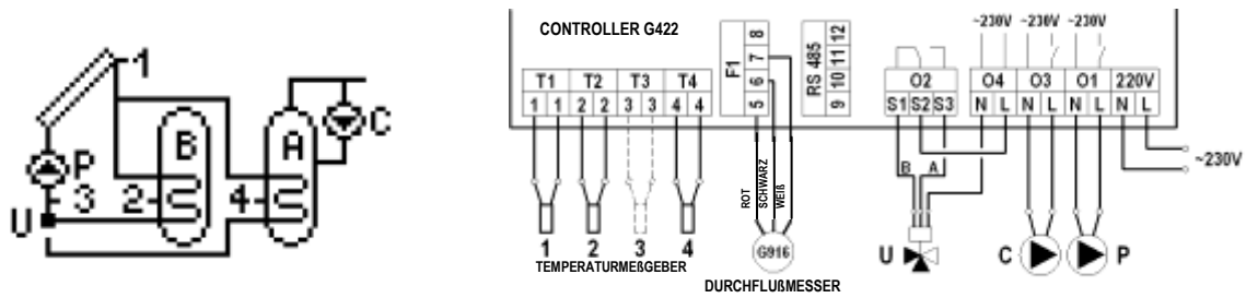
Abb. 13. Anschluss- und elektrisches Schema der Installation Nr. 11.
