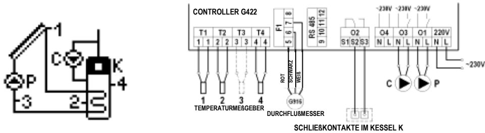
Abb. 7. Anschluss- und elektrisches Schema der Installation 5.
