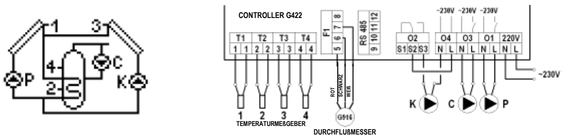
Abb. 17. Anschluss- und elektrisches Schema der Installation 15.
