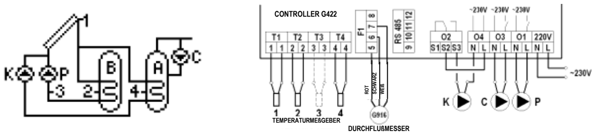
Abb. 14. Anschluss- und elektrisches Schema der Installation Nr. 12.
