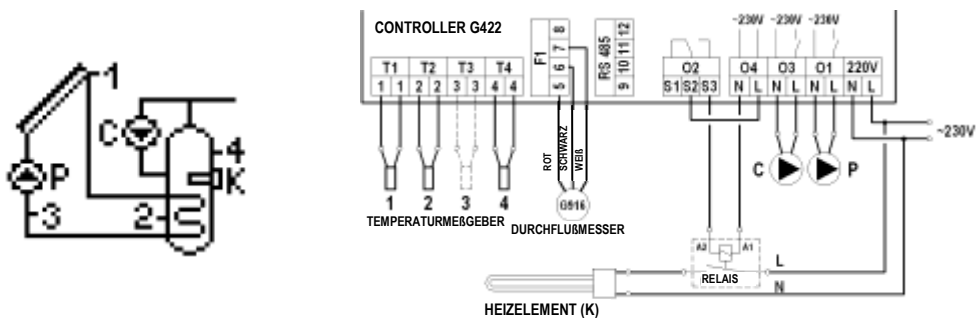
Abb. 6. Anschluss- und elektrisches Schema der Installation 4.
