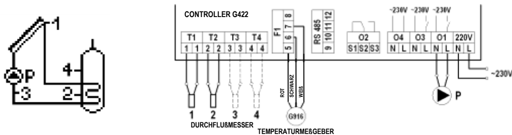
Abb. 3. Anschluss- und elektrisches Schema der Installation 1.
