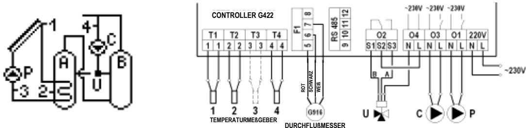
Abb. 10. Anschluss- und elektrisches Schema der Installation Nr. 8.
