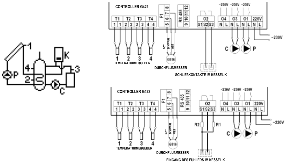
Abb. 16. Anschluss- und elektrisches Schema der Installation Nr.14.
